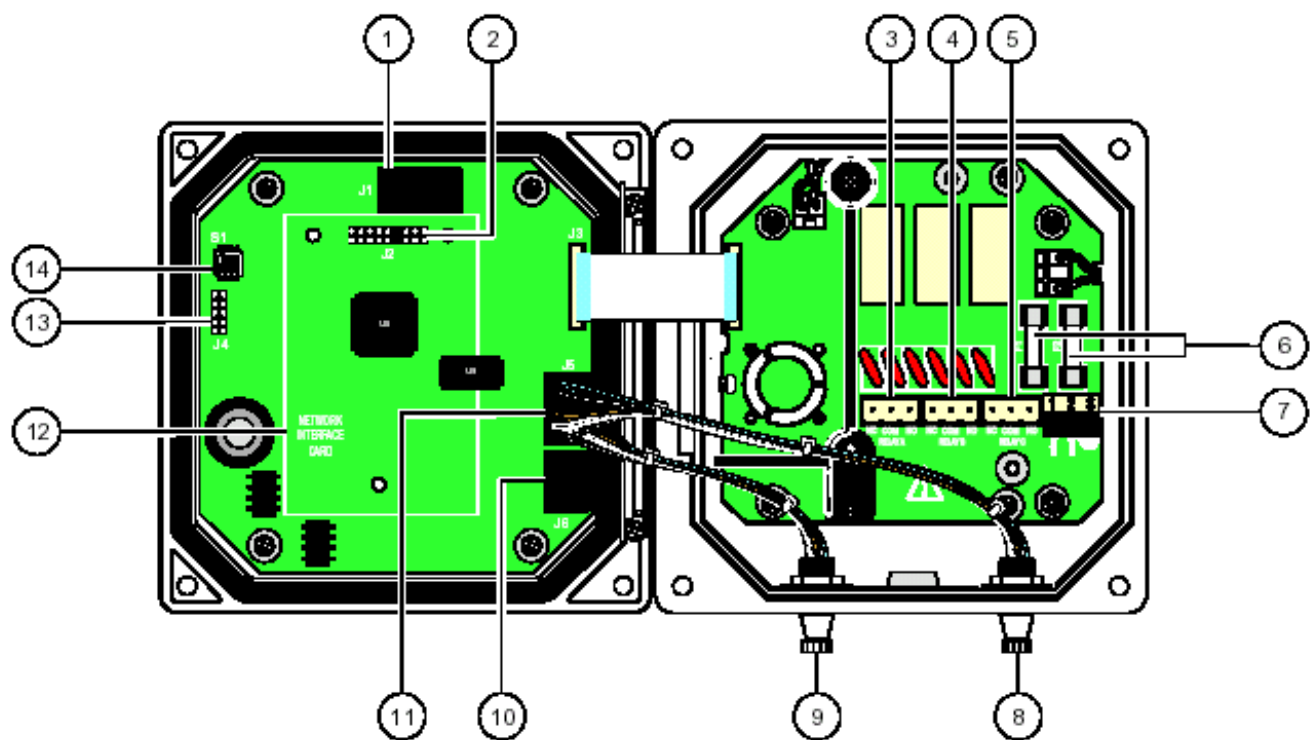
图 15 布线连接
